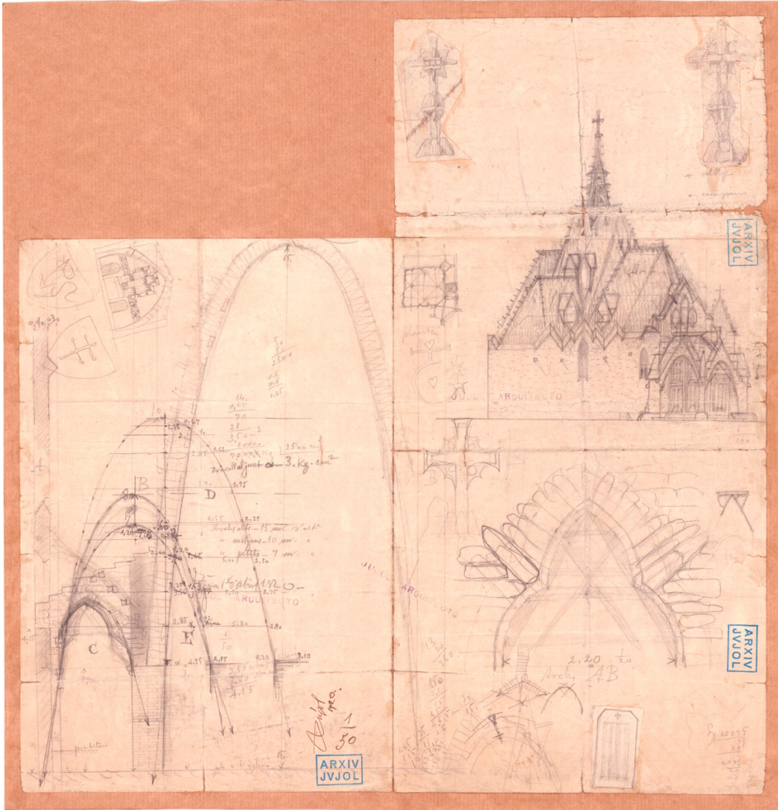
Dibuix dels arcs E 1:50, art trilobulat, 1:20, alçat exterior de l'edifici 1:100, podem datar el dibuix, per la versió de la coberta, del voltant de 1920. (Arxiu Jujol 1854)
